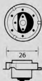
P26s
